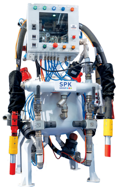
Напорный агрегат непрерывного действия на двух операторов
